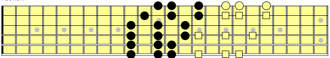
Æolian
